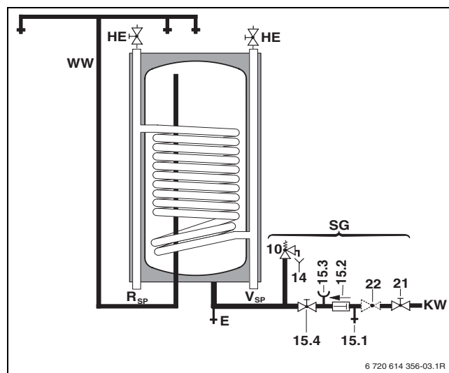
Obr. 5 Schéma zapojení části pro pitnou vodu
